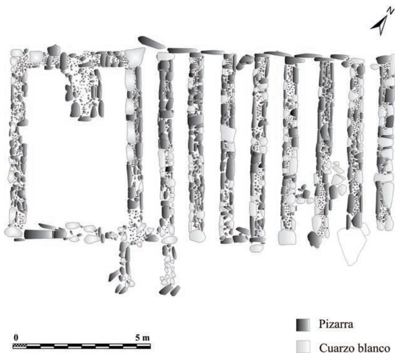
Fig. 4. Pianta dell' horreum della villa romana di Monroy (Cáceres). Immagine: autore.
